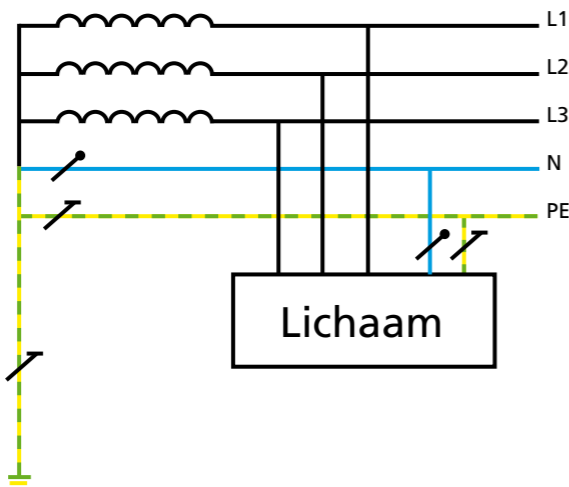
TN-S netwerk: Neutrale geleider en aardingsgeleiding gescheiden
